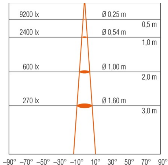
Lichtverteilung
