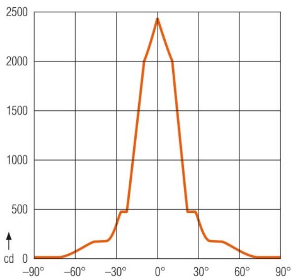
Lichtverteilung
